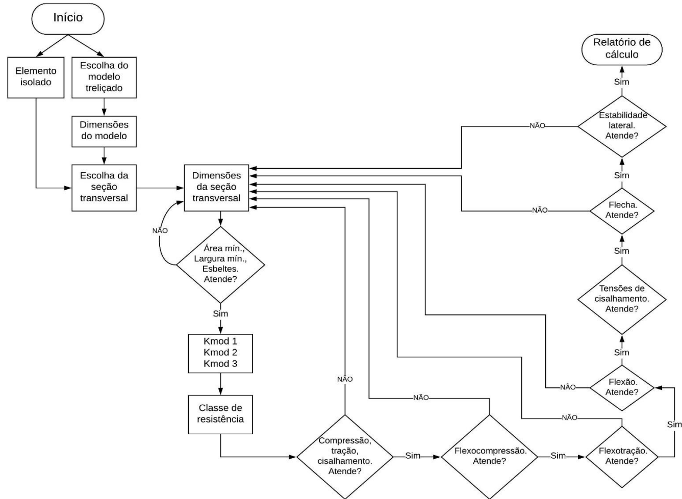
Figura 1 - Fluxograma geral.
